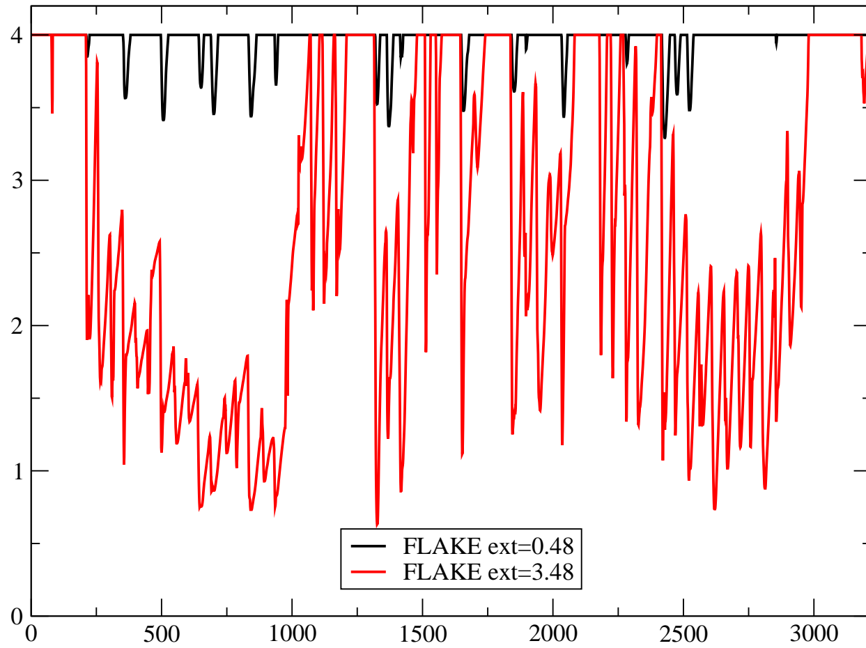
B11 : mixed layer depth
